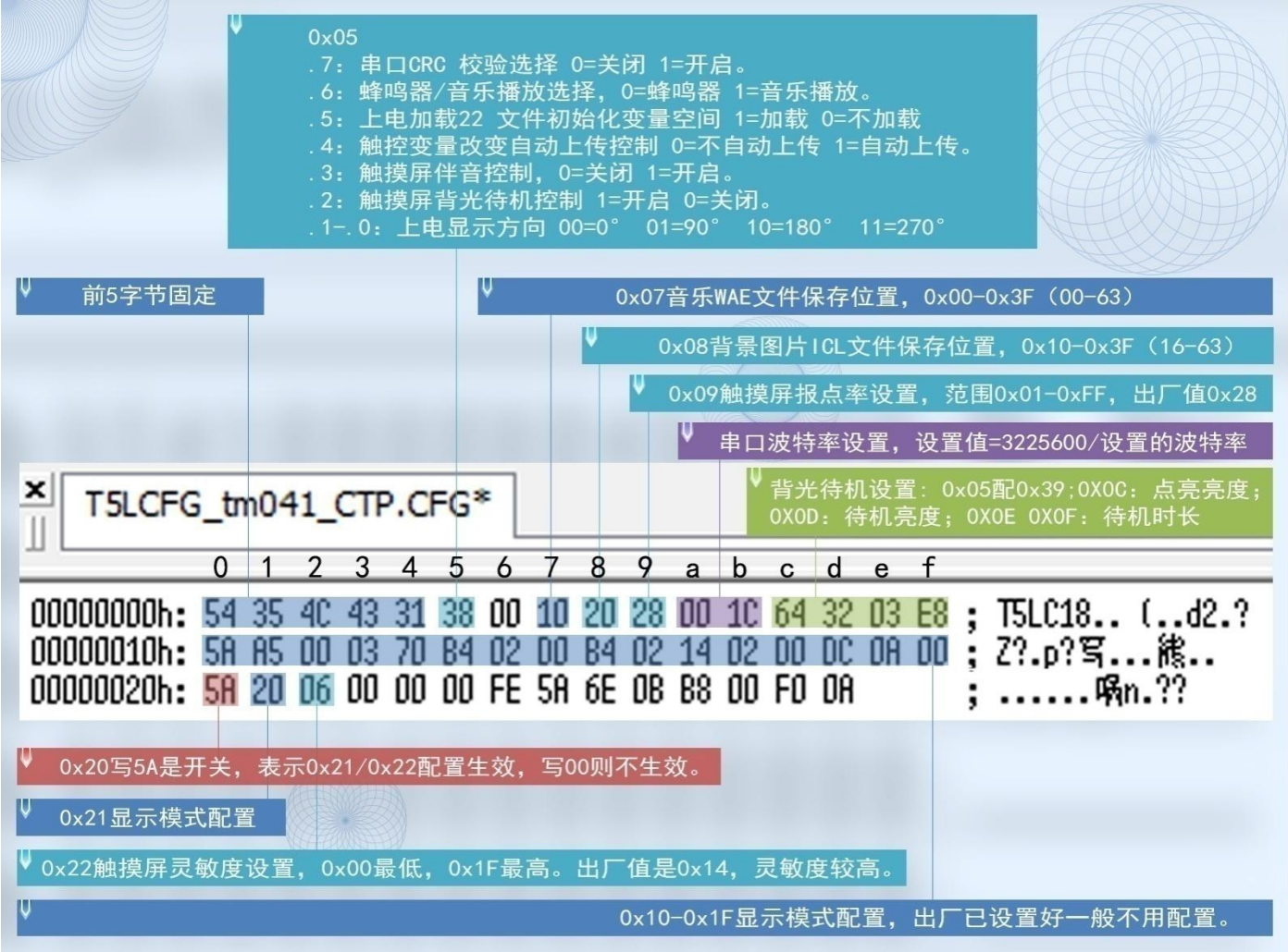
图 3.7 CFG 文件配置总图
