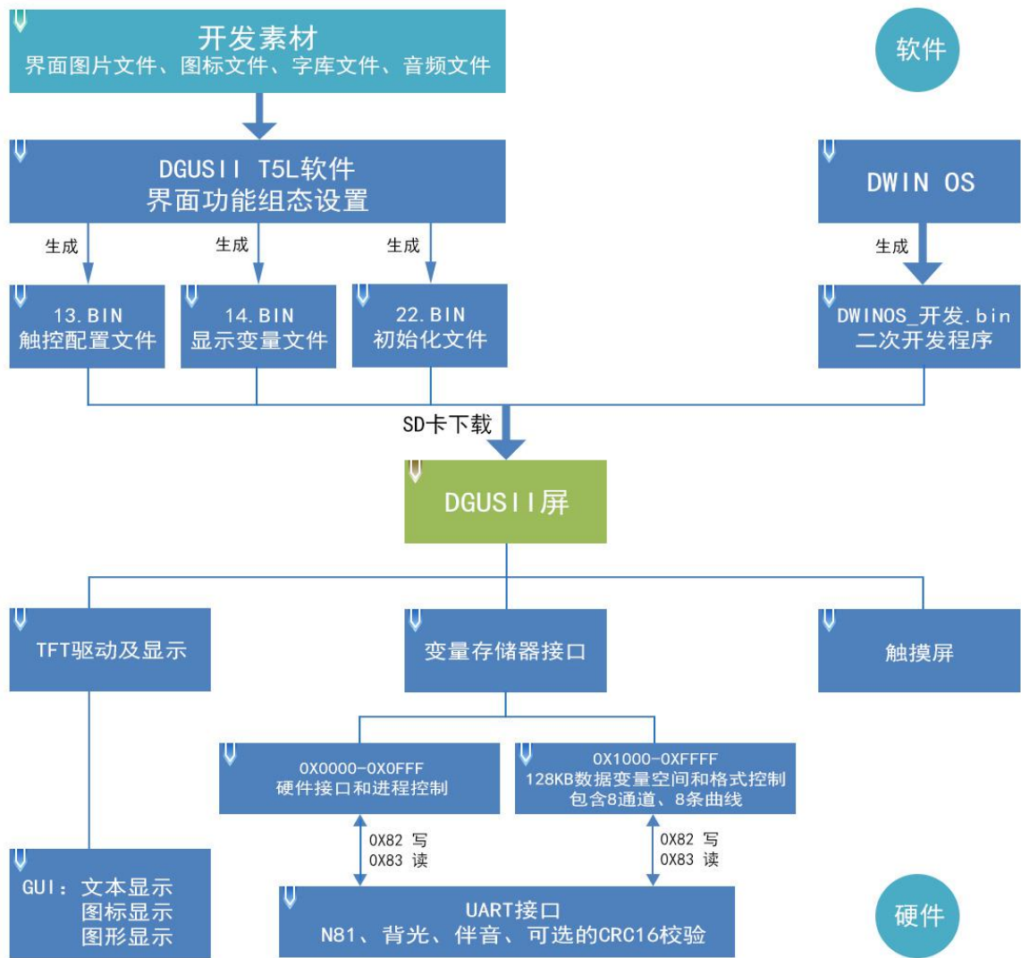
图 2.2T5L_DGUS2 开发体系图解
