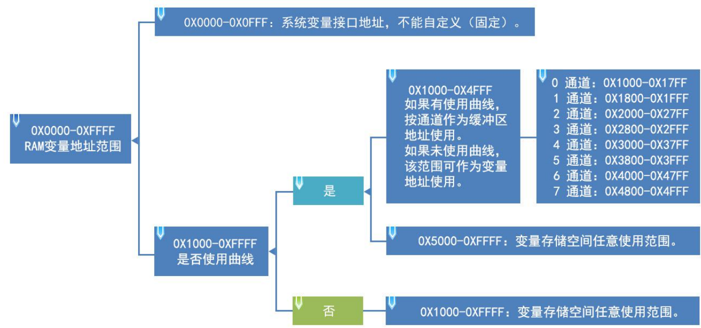
图2.5 RAM存储器空间划分
