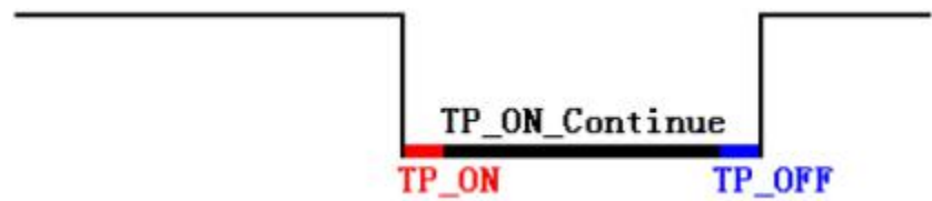
图 6.13 触摸屏按压的 3 个状态
